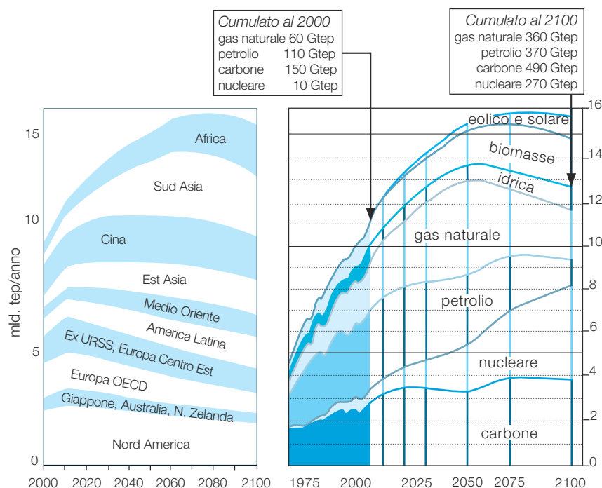
Fig. 4 - SCENARIO STIMATO DEI FABBISOGNI GLOBALI DI ENERGIA PER IL XXI SECOLO (1)
