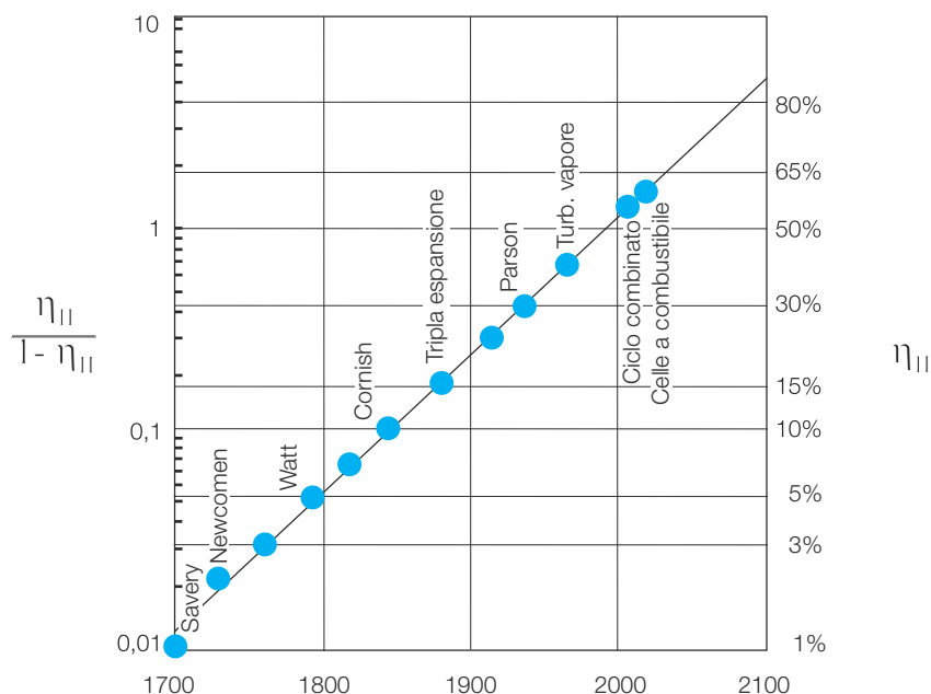
Fig. 1 - EVOLUZIONE DELL'EFFICIENZA TERMODINAMICA DI SECONDO PRINCIPIO DELLE MACCHINE DI CONVERSIONE DELL'ENERGIA NEGLI ULTIMI 300 ANNI
