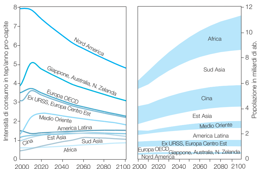
Fig. 3 - PREVISIONE DI CRESCITA DEMOGRAFICA PER IL XXI SECOLO (A DESTRA) E DI VARIAZIONE DEI CONSUMI PRO-CAPITE (A SINISTRA) PER GRUPPI DI NAZIONI OMOGENEE PER TIPO DI ECONOMIA E DI LIVELLO DI SVILUPPO INDUSTRIALE
