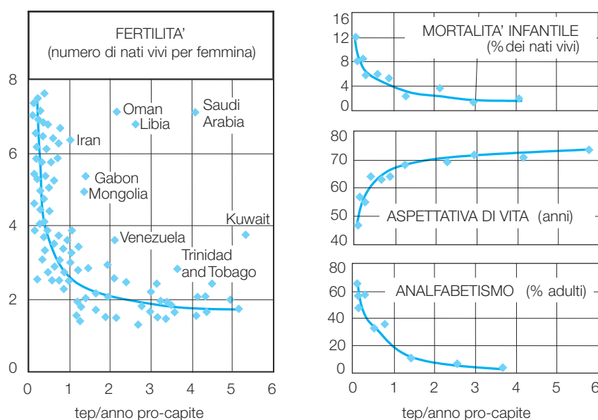
Fig. 2 - CORRELAZIONI FRA DIVERSI INDICATORI DI LIVELLO DI SVILUPPO SOCIO-ECONOMICO E CONSUMO PRO-CAPITE DI ENERGIA
